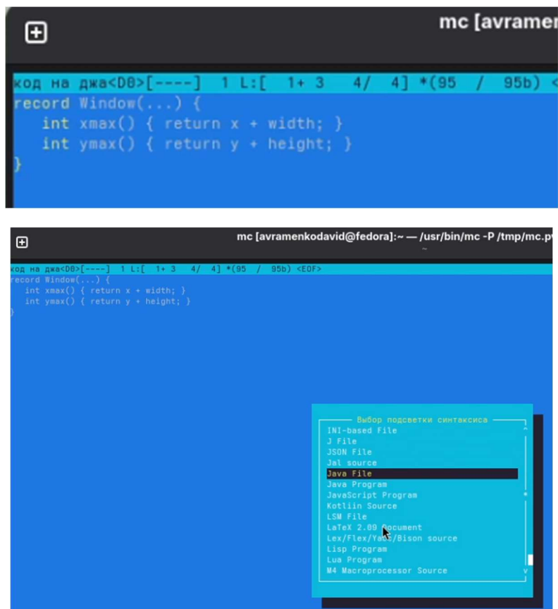
Рисунок 3.23: Включение подсветки синтаксиса
